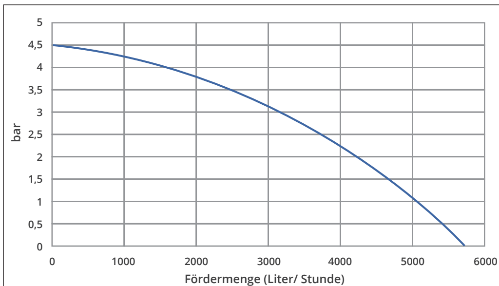
Pumpenkennlinie (Leistungsdiagramm)
