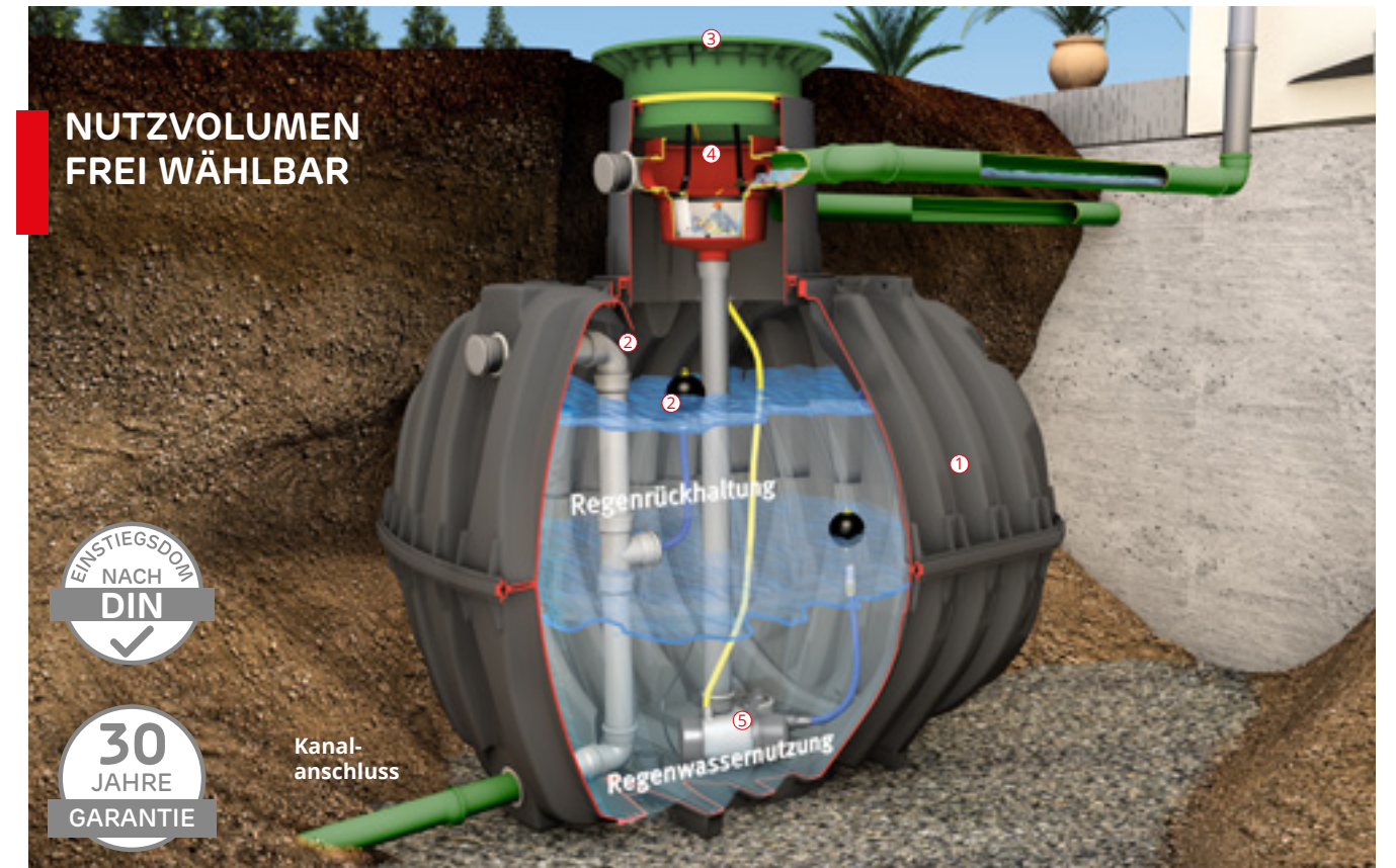
Abb. zeigt Carat Retentionszisterne Plus mit Carat Retention Ausbaupaket 2 (Zubehör unten) und Technikpaket Garten-Komfort (Zubehör Seite 68)
