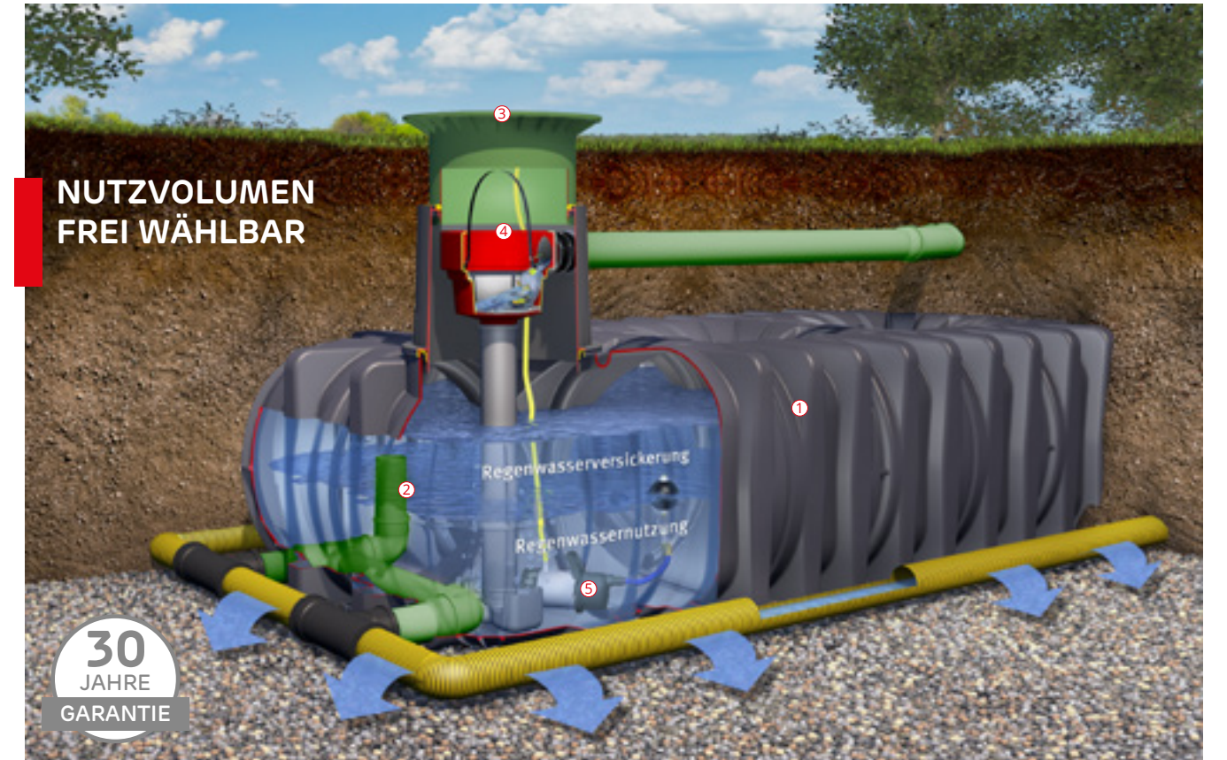
Abb. zeigt Platin XL Versickerung Plus mit Platin XL Retention/Versickerung Ausbaupaket 2 (siehe Zubehör) und Technikpaket Garten-Komfort (Seite 42)
