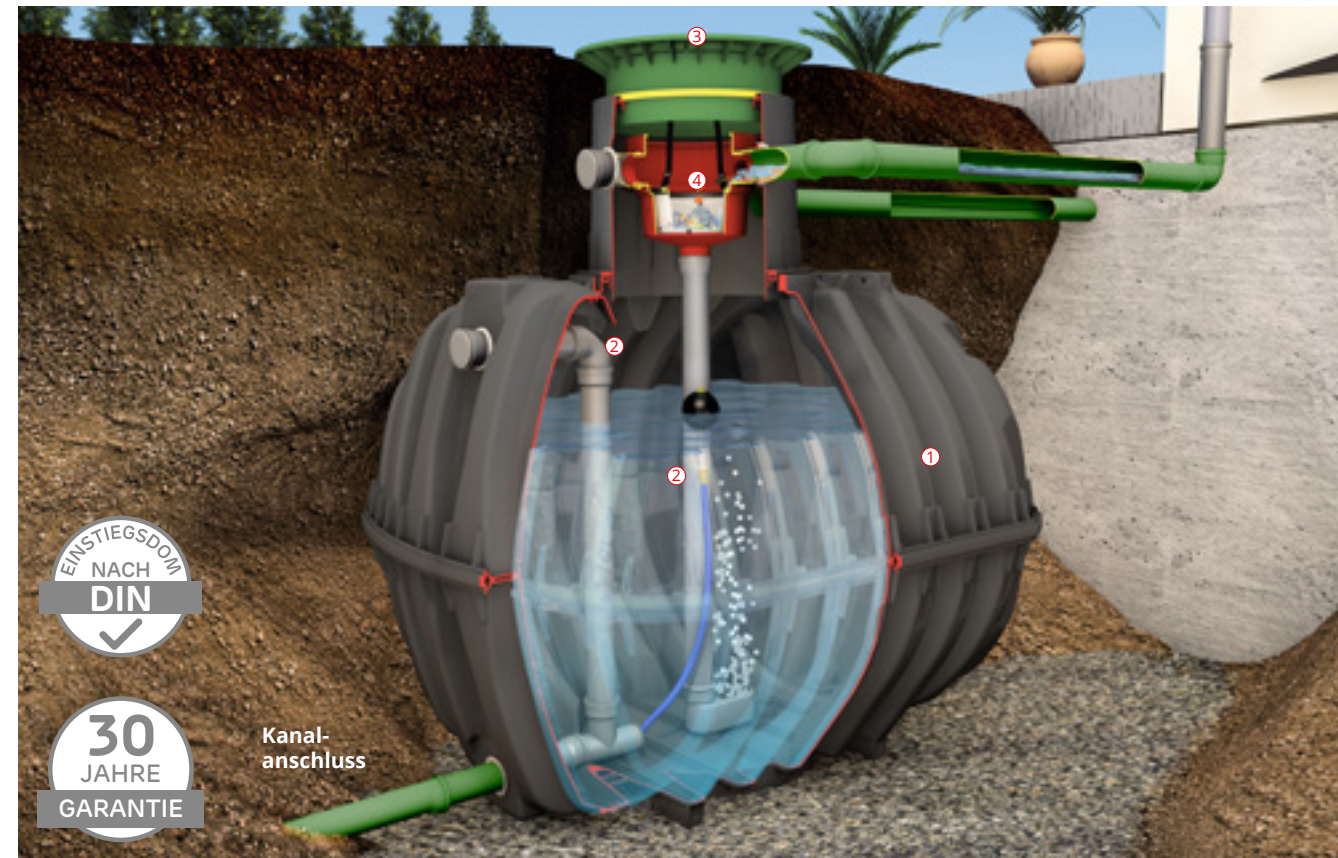
Abb. zeigt Carat Retentionszisterne mit beruhigtem Zulauf (Zubehör Seite 121)
