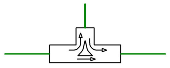
Prinzip Umspülventil
