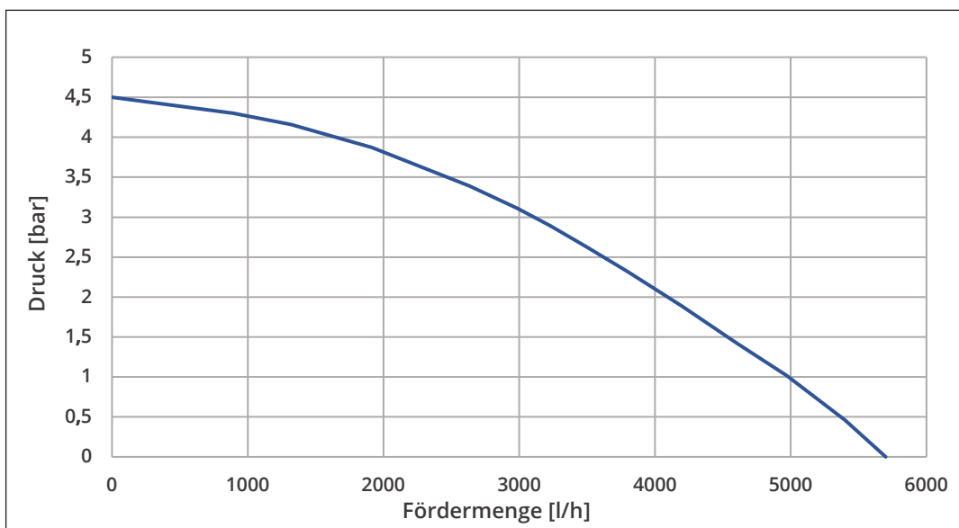
Pumpenkennlinie (Leistungsdiagramm)
